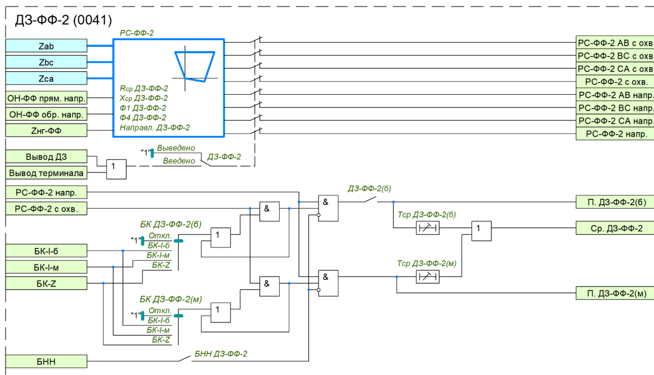
Рисунок 1.8 – Функциональная схема логики ДЗ-FF-2
