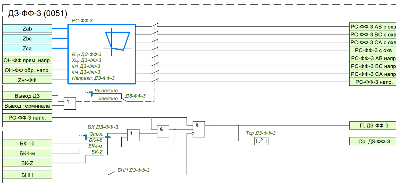
Рисунок 1.9 – Функциональная схема логики ДЗ-FF-3
